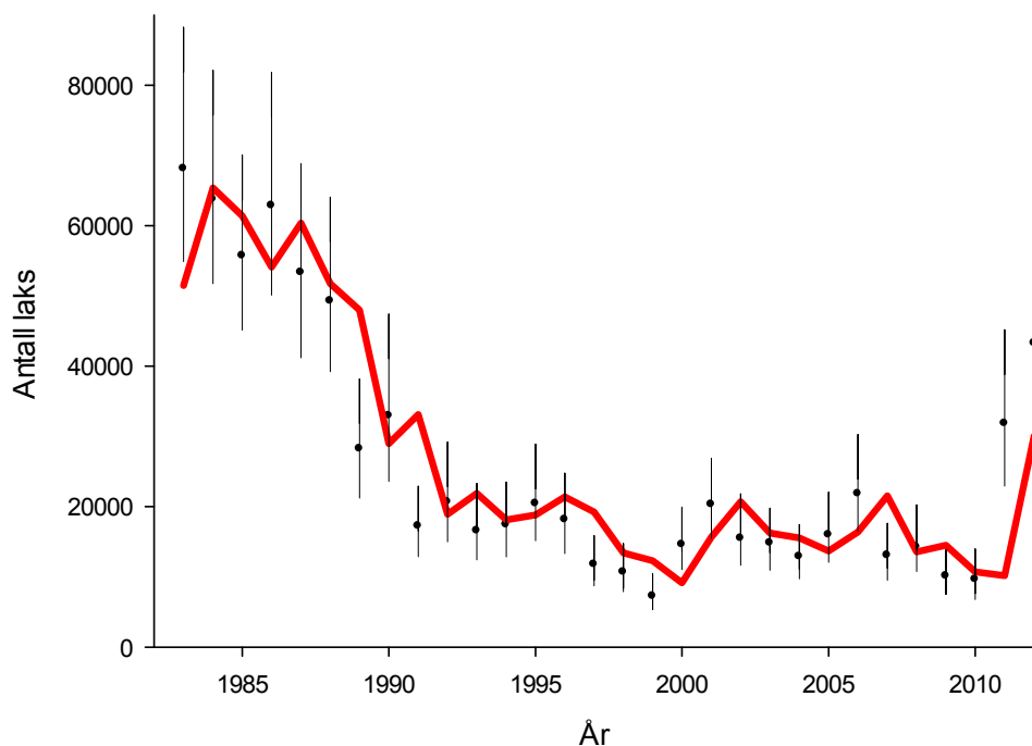
Figur 2.16. Beregnet innsig av mellom- og storlaks (laks <math> > 3 \text{ kg}</math>) til kysten av området fra Hordaland og Sogn og Fjordane i perioden 1983-2012. Punktene angir medianverdiene, mens de lodrette strekene angir spennet mellom minste og største verdi fra simuleringene. Den røde linjen er trendlinjen beregnet fra ARIMA (1,0,0) trendanalysemodell ( R^2 modell = 0,79).
