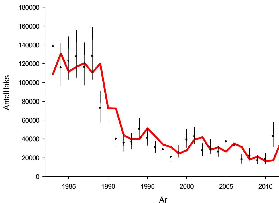
Figur 2.14. Beregnet innsig av alle størrelsesgrupper av laks til kysten av området fra Hordaland og Sogn og Fjordane i perioden 1983-2012. Punktene angir medianverdiene, mens de lodrette strekene angir spennet mellom minste og største verdi fra simuleringene. Den røde linjen er trendlinjen beregnet fra ARIMA (1,0,0) trendanalysemodell ( R^2_{modell} = 0,83 ).
